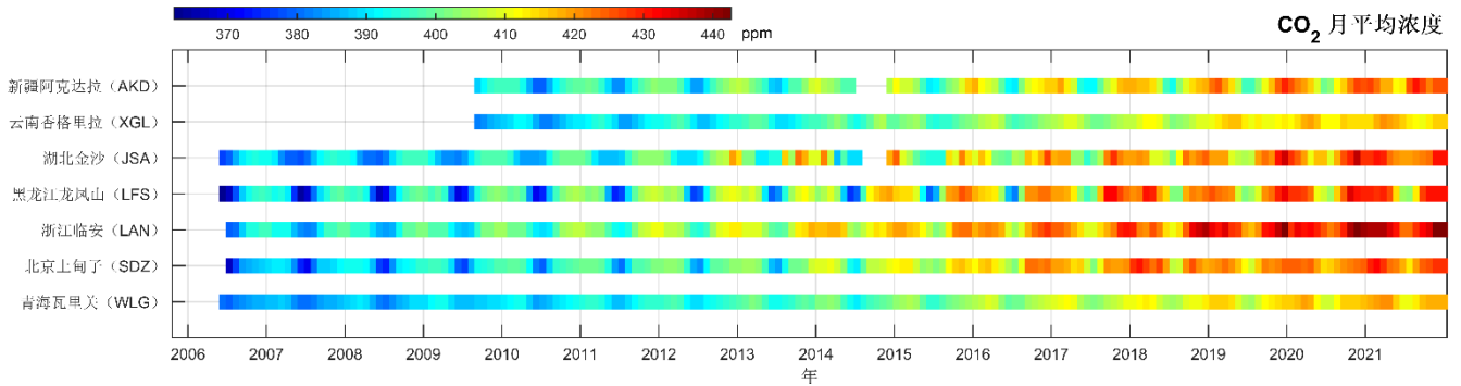
图2 中国气象局7个大气本底站2006~2021年大气CO 2 逐月平均浓度
