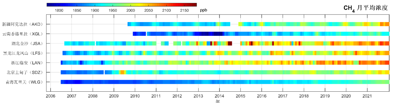
图3 中国气象局7个大气本底站2006~2021年大气CH 4 逐月平均浓度
