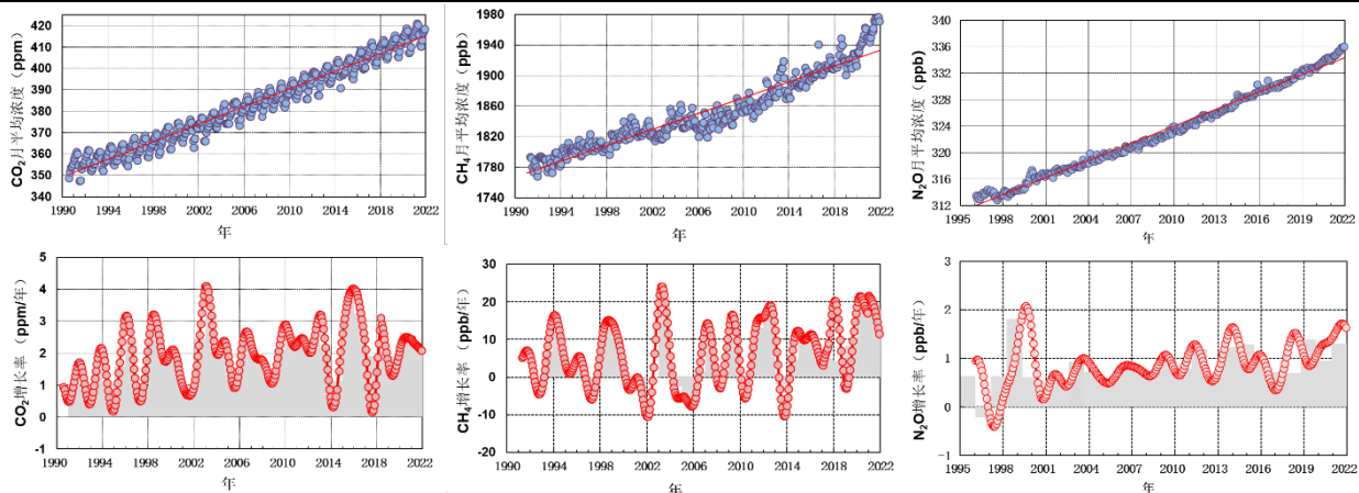
图1 1990年以来瓦里关站大气CO 2 、CH 4 、N 2 O浓度（上图）及其增长率（下图）
